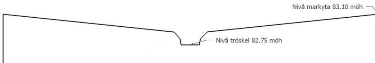
Principskiss
